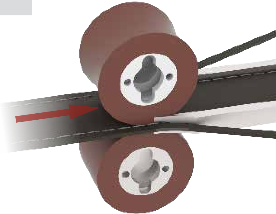
RULLI DI RIFILATURA TRIMMING ROLLERS
